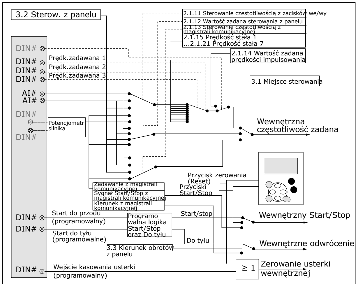
Rys. 18: Logika sygnału sterowania aplikacji sterowania uniwersalnego
