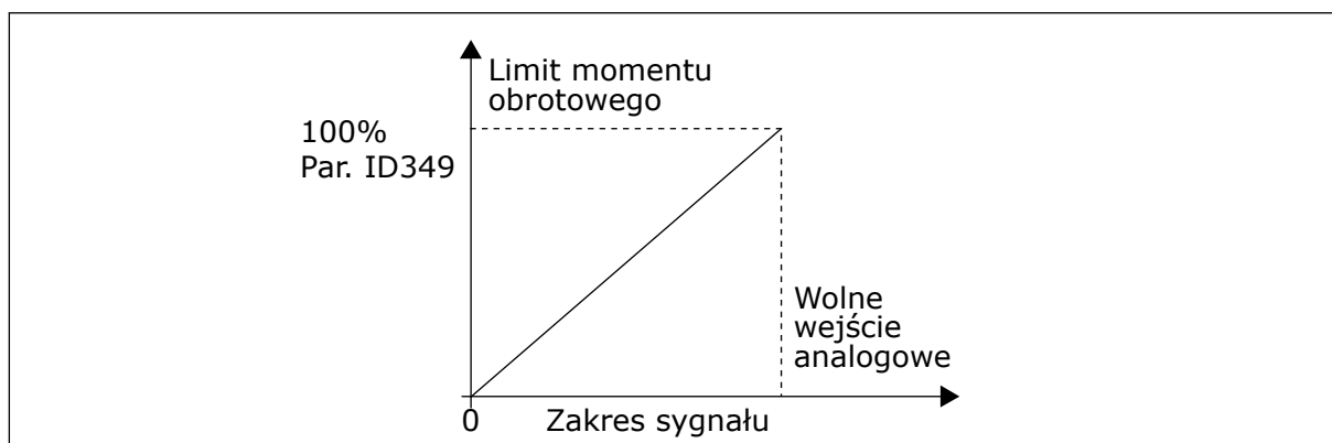
Rys. 53: Zmniejszenie limitu monitorowania momentu obrotowego
