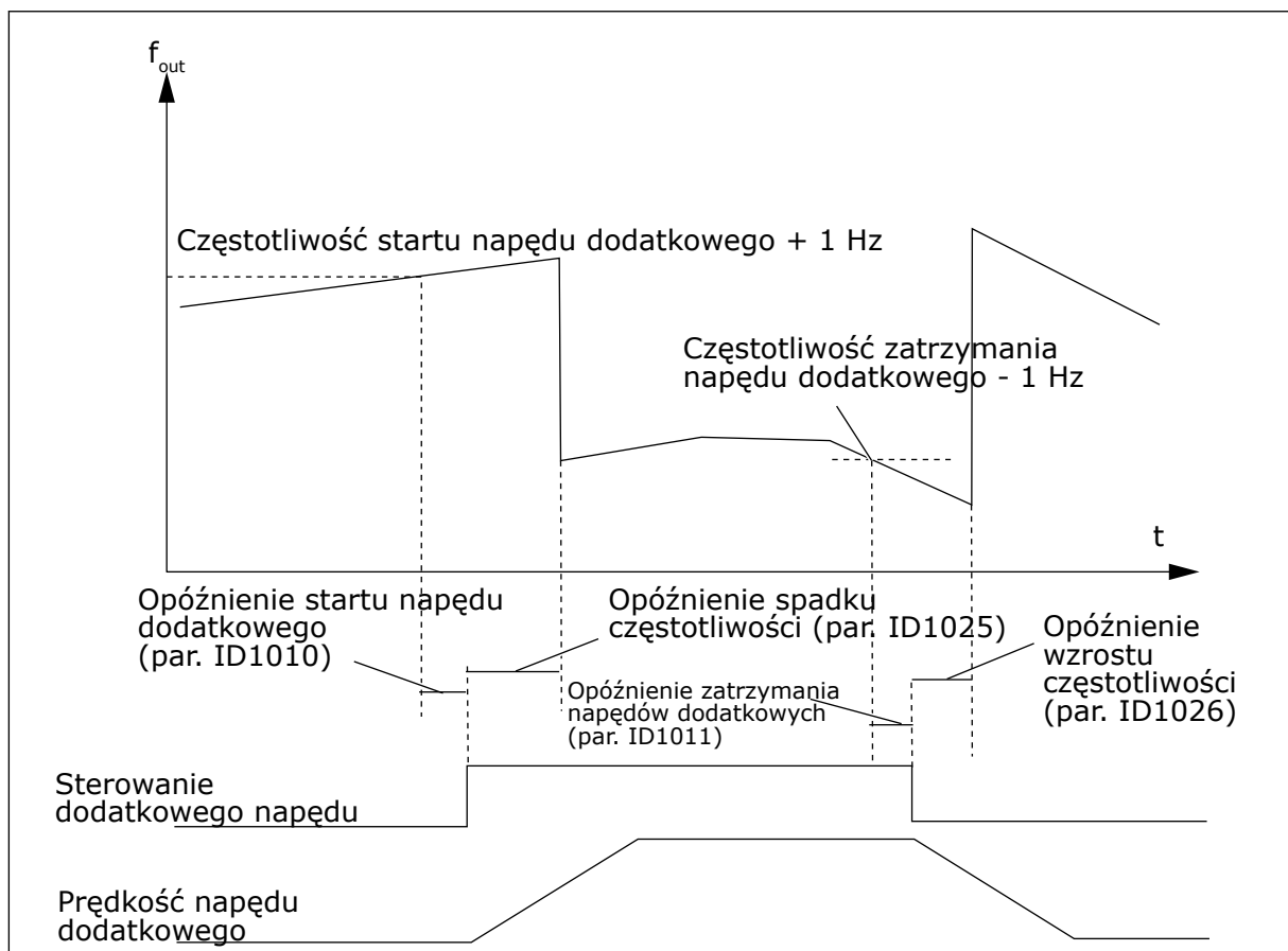
Rys. 85: Opóźnienia spadku i wzrostu częstotliwości
