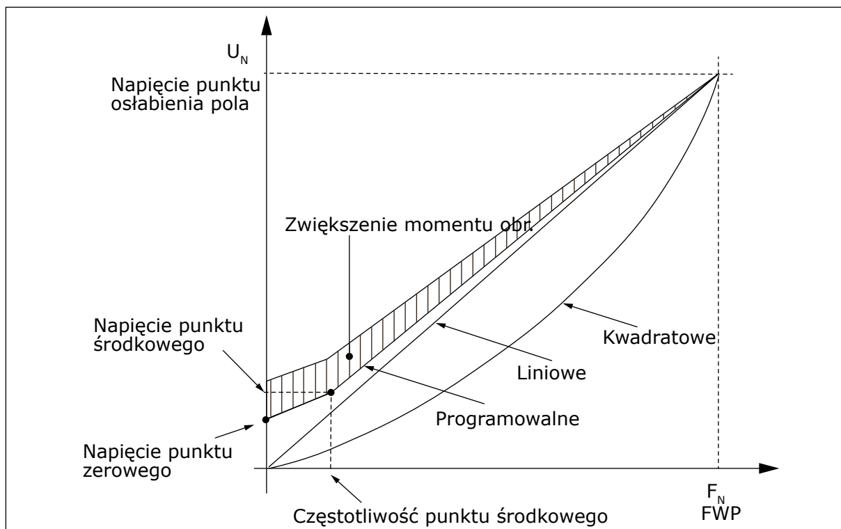
Rys. 26: Optymalizacja U/f
